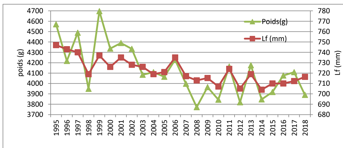
Fig. 8 : Evolution des tailles et poids moyens des saumons de printemps piégés au Moulin des Princes de 1995 à 2018
