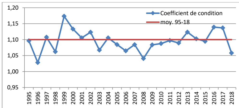
Fig. 9 : Evolution des coefficients de condition des saumons de printemps piégés au Moulin des Princes de 1995 à 2018
