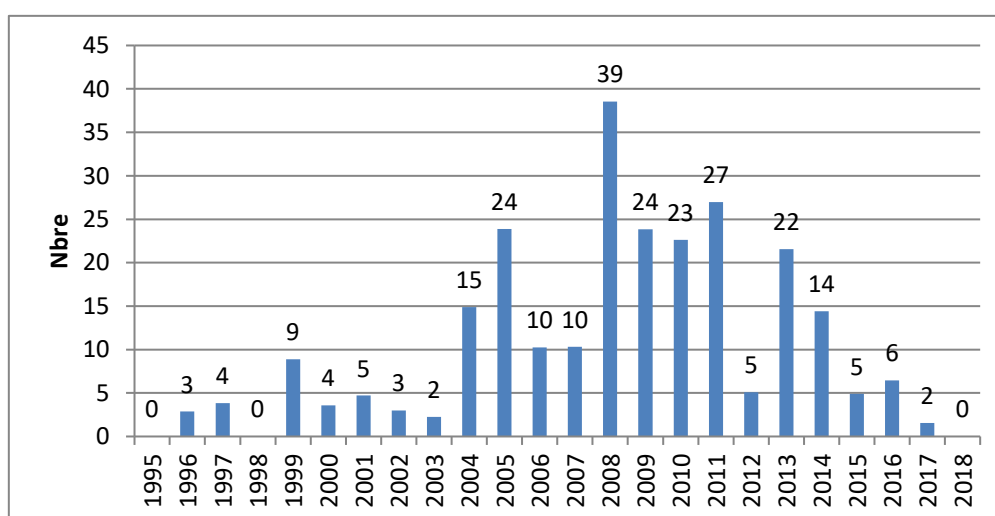
Fig. 6 : Evolution du nombre de saumons de 2 nd retour piégés au Moulin des Princes de 1995 à 2018
